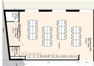
Konferenzbestuhlung 48 Sitzplätze
